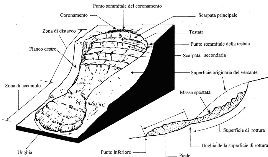
Figura 2-7 - Nomenclatura delle frane (Varnes 1978)
